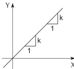
Figura 13: Curva que representa la función y = kx . En cualquier parte de la curva (recta), por cada unidad que varía la variable independiente, la variable dependiente varía k unidades.
