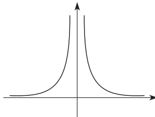
Figura 15: Curva que representa la función y = k/x^2 . Cerca del cero, los valores de y crecen muy rápidamente, teniendo a + infinito. Conforme la x es muy grande, la función prácticamente no crece (ni decrece). Para los valores negativos de x , la curva es simétrica respecto al eje Y .
