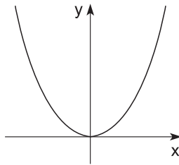
Figura 14: Curva que representa la función y = kx^2 . Cerca del cero, la función crece muy lentamente. Conforme mayor es la x la función crece cada vez más rápidamente. Para los valores negativos de X , la curva es simétrica respecto al eje Y .
